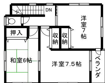
2階間取図
